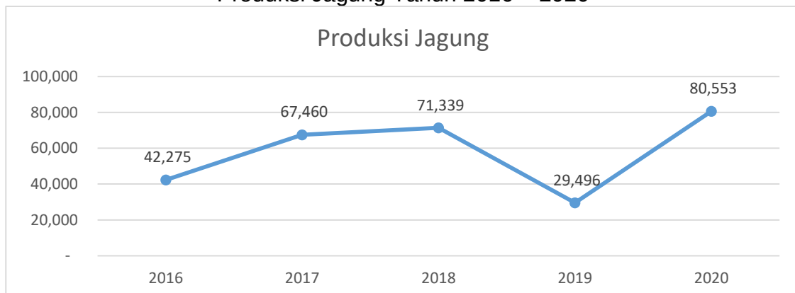
Grafik 2.45 Produksi Jagung Tahun 2016 – 2020
