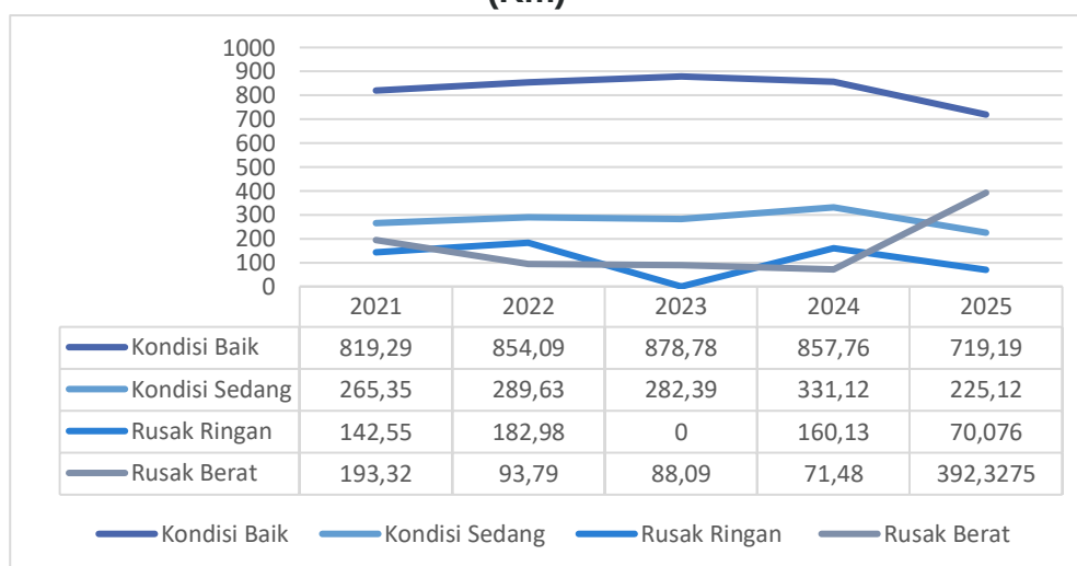
Grafik 3.8 Capaian Kinerja Jalan Kabupaten Musi Rawas Tahun 2021 – 2025 (Km)
